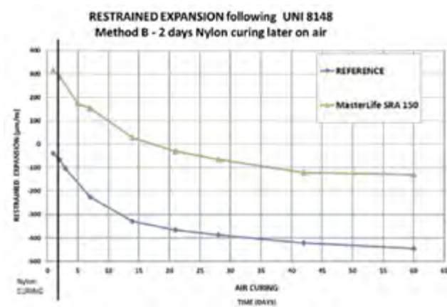
Rys. 1. Redukcja skurczu betonu dzięki MasterLife SRA 150. CEM I 42,5 R= 300 kg/m 3 , woda= 180 kg/m 3 , kruszywo 1975 kg/m 3 , MasterLife SRA 150= 20 kg/m 3 .
